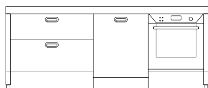
Elemento con pannello per lavastoviglie e forno da 60 cm Element with dishwasher panel and oven 60 cm wide
