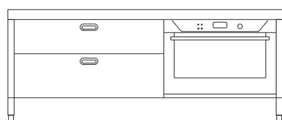
Elemento per forno da 90 cm Element for oven 90 cm wide
